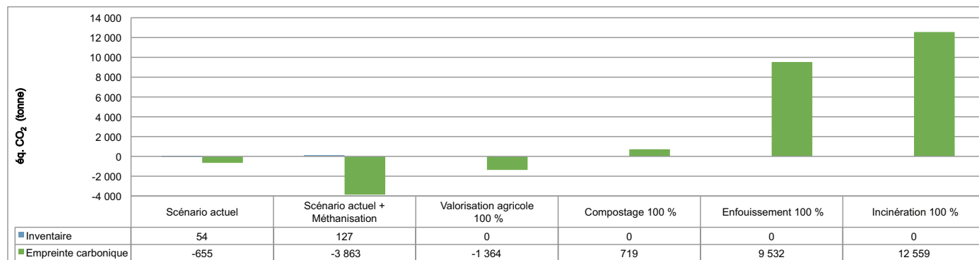
Figure 2 : Comparaison des émissions annuelles de la gestion des biosolides de Saguenay pour tous les scénarios
